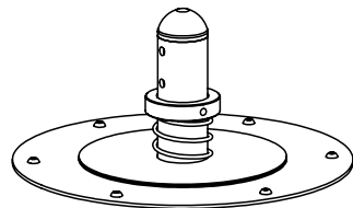
Skizze 4b: Regenschutz
