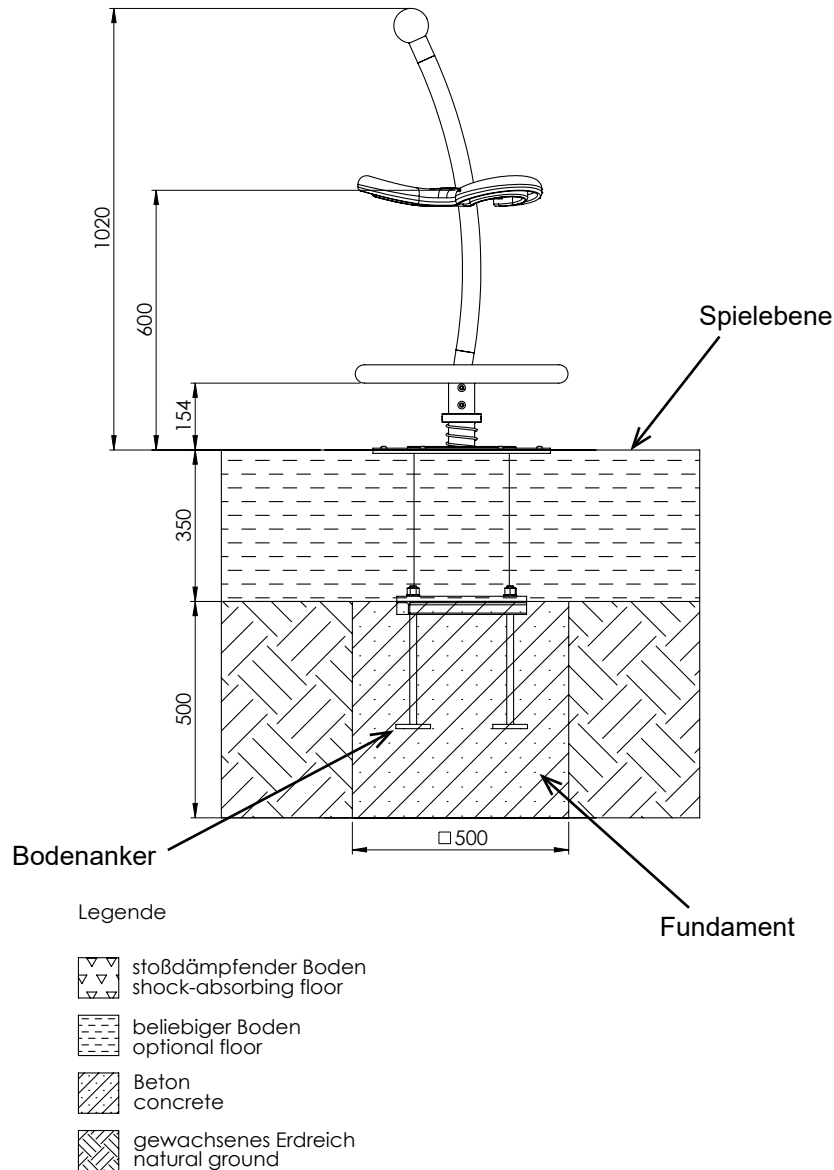
Skizze 2: Fundamentplan
