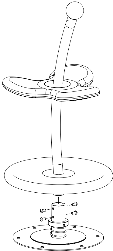
Skizze 4a: Vorübergehende Demontage
